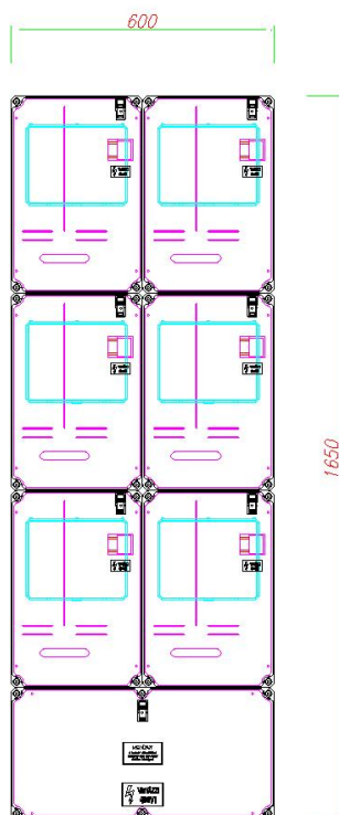
KÖRVONALRAJZ (méretezett):
